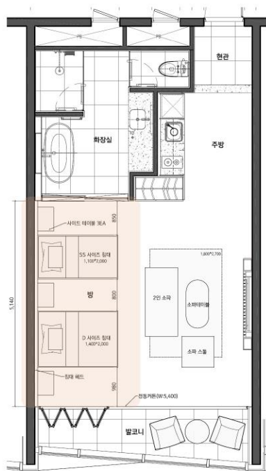
▲ 평면도
